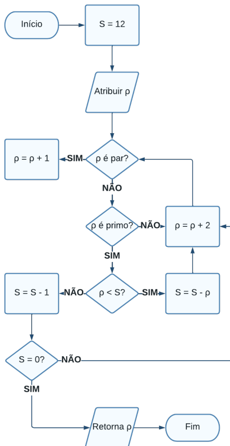
Fluxograma 1 – Exemplo de fluxograma de algoritmo
