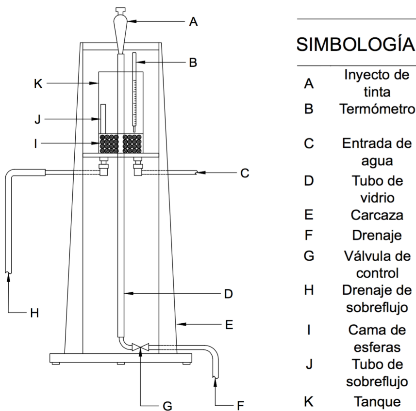
Figura 2.1. Equipo de determinación del número de Reynolds utilizado en el laboratorio de Ingeniería Civil. (Fuente: Elaboración propia)
